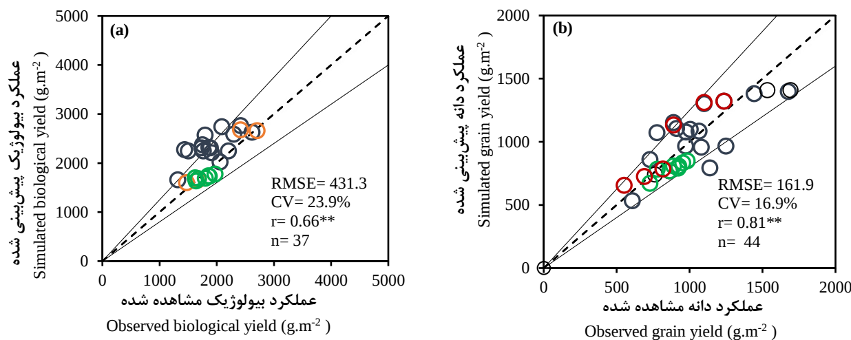
شکل ۳- عملکرد بیولوژیک (a) و عملکرد دانه (b) شبیه‌سازی شده در مقابل مشاهده شده دامنه \pm 20\% درصد اختلاف بین داده‌های شبیه‌سازی و مشاهده شده با خطوط ممتد و خط ۱:۱ به صورت با خط نقطه‌چین نشان داده شده است. همچنین ** نشان دهنده معنی داری در سطح یک درصد است.
