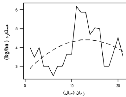
شکل ۲: روند ۲۰ ساله عملکرد زعفران در تربت حیدریه.
