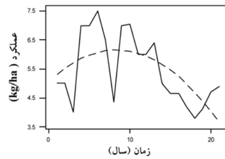
شکل ۴: روند ۲۰ ساله عملکرد زعفران در بیرجند.
