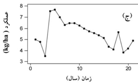
شکل ۳: الف) روند تغییرات عملکرد زعفران در بیرجند در طی ۲۰ سال گذشته، ب) تغییرات فصلی عملکرد زعفران در طی بیست سال گذشته با حذف روند از داده‌ها، ج) تصحیح داده‌های عملکرد زعفران در بیست سال گذشته.
