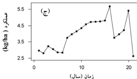
شکل ۱: الف) روند تغییرات عملکرد زعفران در تربت حیدریه در طی ۲۰ سال گذشته، ب) تغییرات فصلی عملکرد زعفران در طی بیست سال گذشته با حذف روند از داده‌ها، ج) تصحیح داده‌های عملکرد زعفران در بیست سال گذشته.
