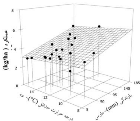
شکل ۵: رابطه بارندگی ماه مارس و درجه حرارت حداقل ماه مه با عملکرد
