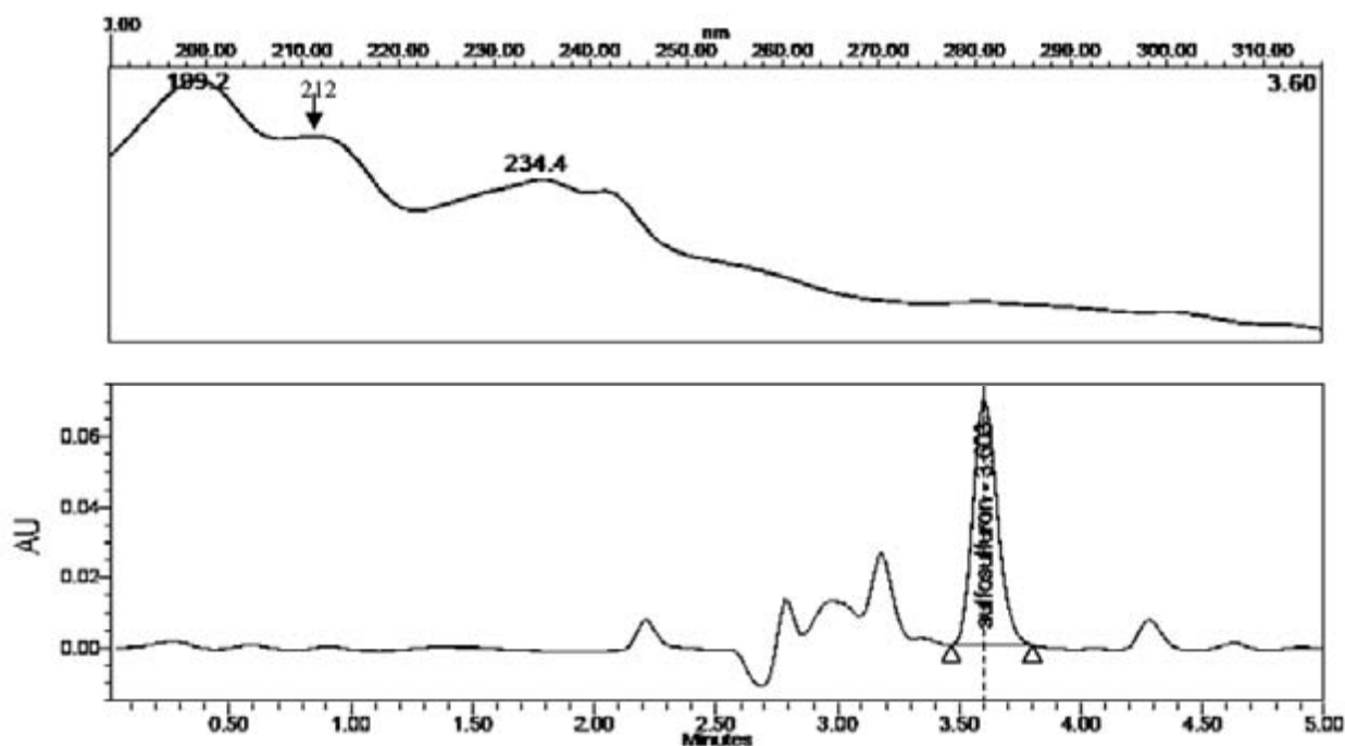
شکل ۱: جذب طیف ماورای بنفش برای سولفوسولفورون (بالا) و کروماتوگرام حاصله (پایین) در آن طیف برای 5 \mu\text{g mL}^{-1} محلول استاندارد (زمان بازداری ۳/۶ دقیقه).
