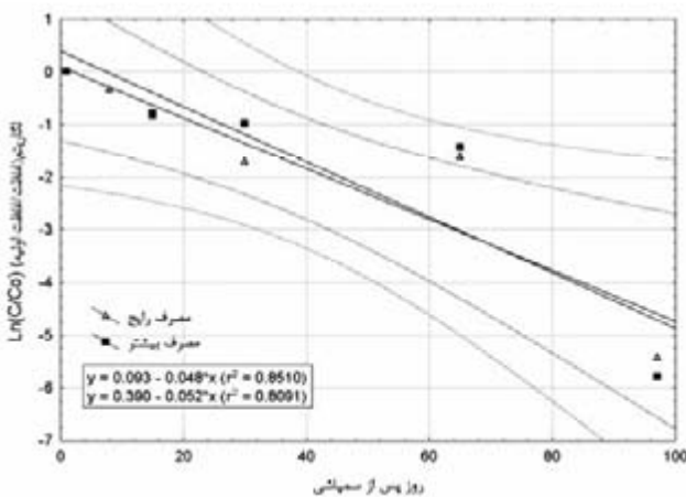
شکل ۲: روند کاستی سم در برابر زمان در خاک بدون کود حیوانی (بالا) و خاک حاوی کود حیوانی (پایین)، فواصل اطمینان ۹۵٪ برای هر خط رگرسیون به شکل خطوط نقطه چین در شکل نشان داده شده است.
