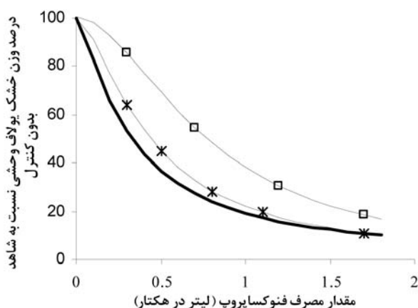
شکل ۶: درصد وزن خشک علف‌هرز یولاف وحشی به مقادیر مختلف علف‌کش فنوکسپروپ‌پی‌اتیل شرکت گل‌سم (□) شرکت گیاه (×) و شرکت بیسترفلد (—) ۳۰ روز پس از سمپاشی در آزمایش گلخانه‌ای.
