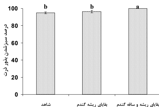
شکل ۱- اثر سطوح بقایای گندم بر درصد سبزشدن بذور ذرت. ستون‌های داری حرف مشترک از لحاظ آماری در سطح احتمال ۵ درصد اختلاف معنی‌داری ندارند (آزمون دانکن). میله‌های عمودی نشان‌دهنده خطای استاندارد (SE) در هر تیمار می‌باشند.
