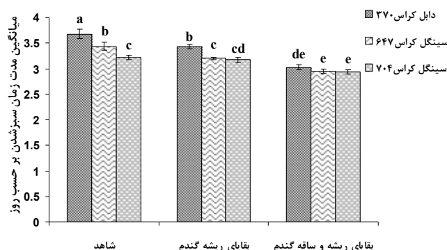
شکل ۲- اثر متقابل رقم و سطح بقایای گندم بر میانگین مدت زمان سبز شدن ذرت. ستون‌های داری حرف مشترک از لحاظ آماری در سطح احتمال ۵ درصد اختلاف معنی‌داری ندارند (آزمون دانکن). میله‌های عمودی نشان‌دهنده خطای استاندارد (SE) در هر تیمار می‌باشند.
