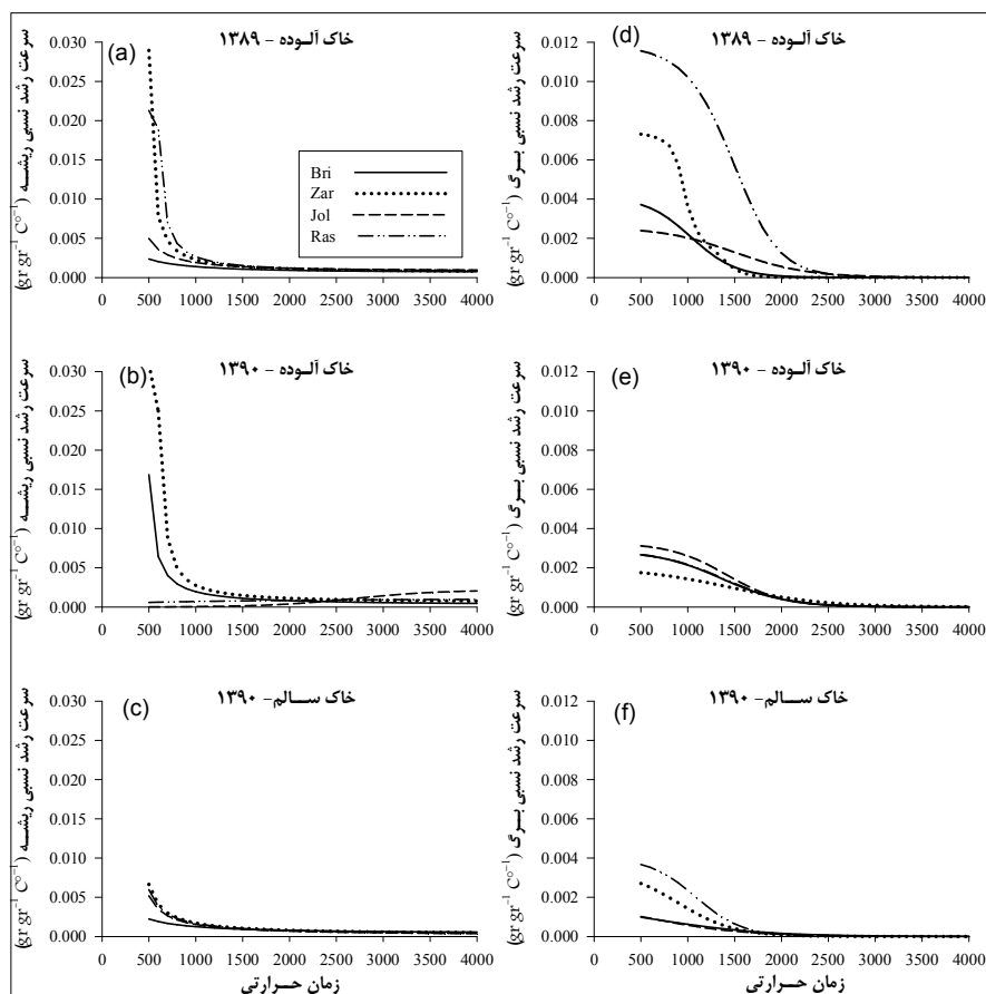
شکل ۷- برازش معادله سرعت رشد نسبی ریشه ذخیره ای (a, b, c) و برگ (d, e, f) (گرم در گرم در واحد حرارتی) ارقام چغندر قند بر اساس زمان حرارتی در خاک آلوده سال های ۱۳۸۹ و ۱۳۹۰ و خاک سالم در سال ۱۳۹۰
