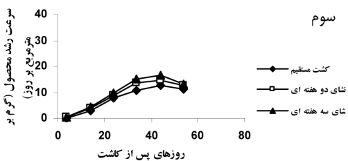
شکل ۲- بررسی اثر تاریخ‌های کاشت اول، دوم و سوم بر سرعت رشد محصول (CGR)
