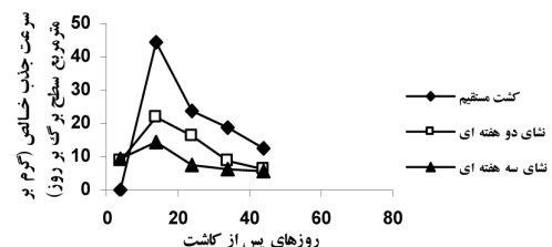
شکل ۳- بررسی اثر تاریخ‌های کاشت اول، دوم و سوم بر سرعت جذب خالص (NAR)
