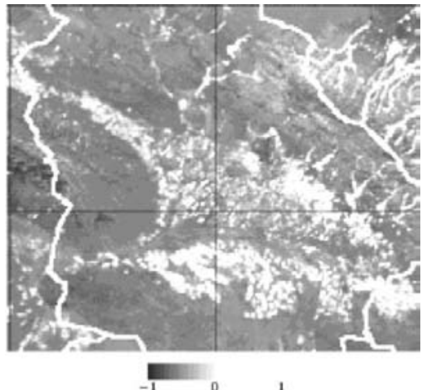
شکل ۱: شاخص NDVI استخراج شده از تصاویر MODIS در منطقه عمومی مورد مطالعه.
