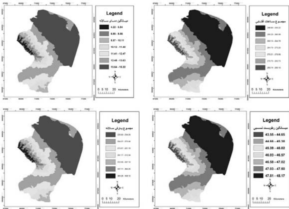
شکل ۲: نقشه‌های پهنه بندی عناصر هواشناسی با استفاده از مدل ارتفاع رقومی:
