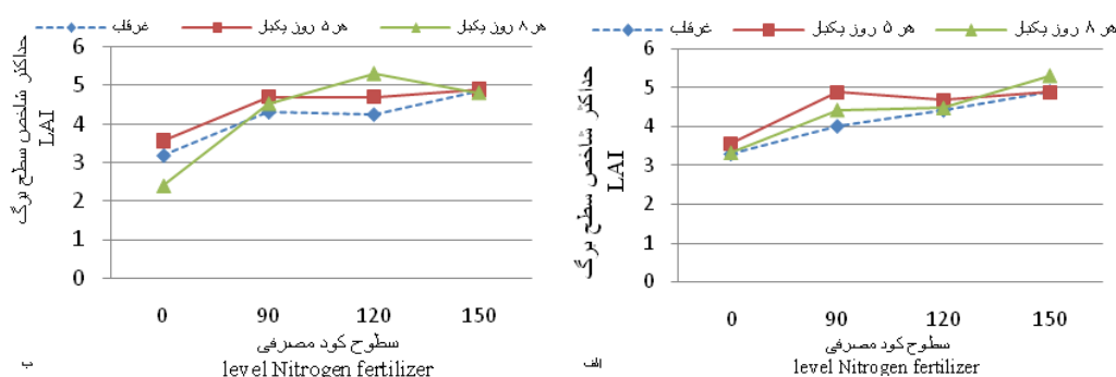
شکل ۴- الف و ب مقادیر شبیه‌سازی شده حداکثر شاخص سطح برگ توسط مدل CropSyst در سطوح آبیاری و کود در سالهای ۱۳۹۲ و ۱۳۹۳ Figure 4- a, b.: Amounts simulated LAI by crowsyst model in levels N & R in year 2013 and 2014
