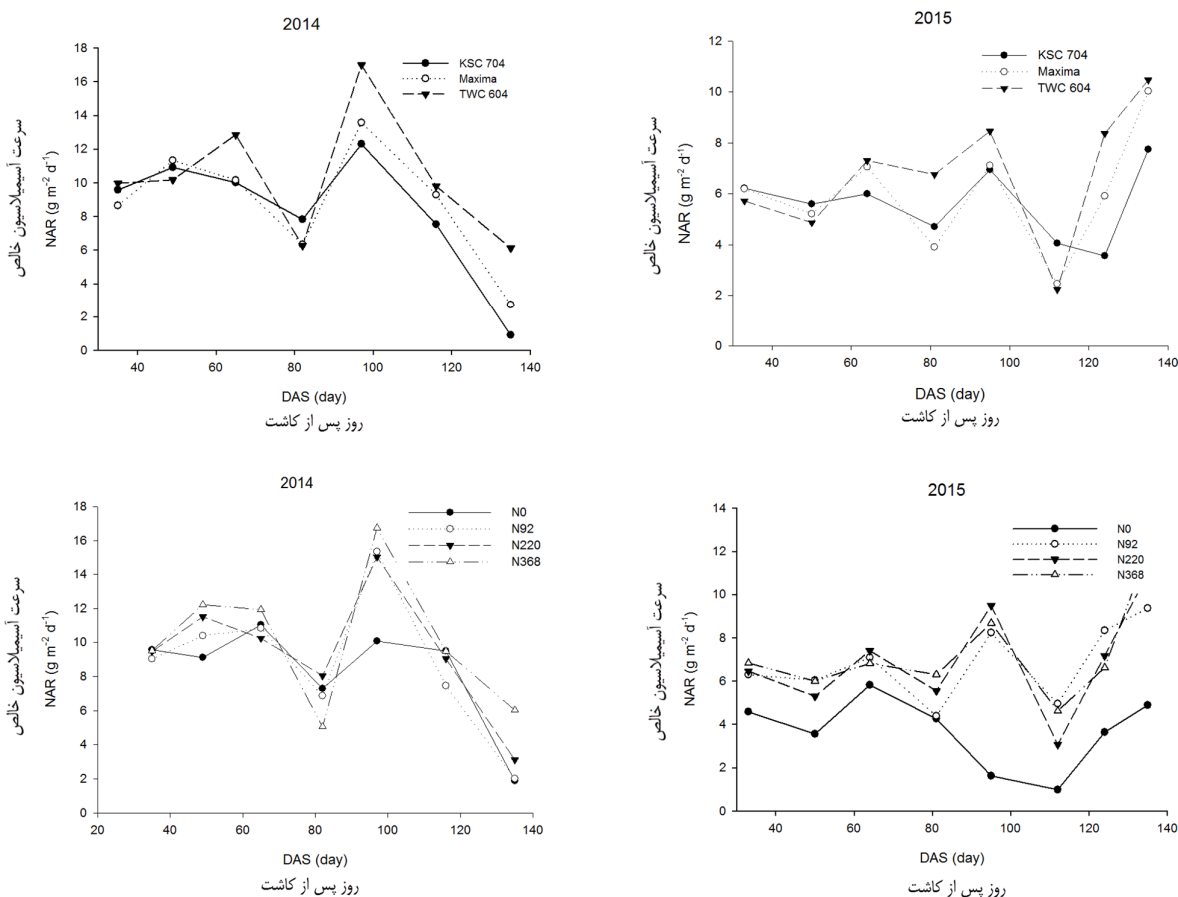
شکل ۳- روند تغییرات سرعت آسیمیلاسیون خالص (NAR) در سه هیبرید ذرت (KSC 704، Maxima و TWC 604) تحت مقادیر مختلف نیتروژن (N0، N92، N220 و N368 کیلوگرم در هکتار) طی سال‌های زراعی ۱۳۹۳ و ۱۳۹۴
